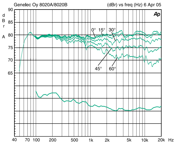
Figur 5. Den övre gruppen av kurvor visar den horisontella riktningskaraktistiken hos 8020B mätt vid 0, 15, 30, 45 samt 60 graders vinkel på 1 m avstånd. Den undre visar systemets effektkurva
